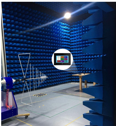
图 7-5 辐射测试图
