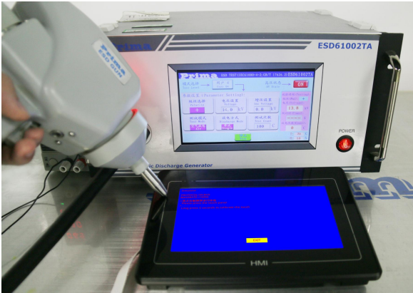
图 7-2 ESD 测试图
