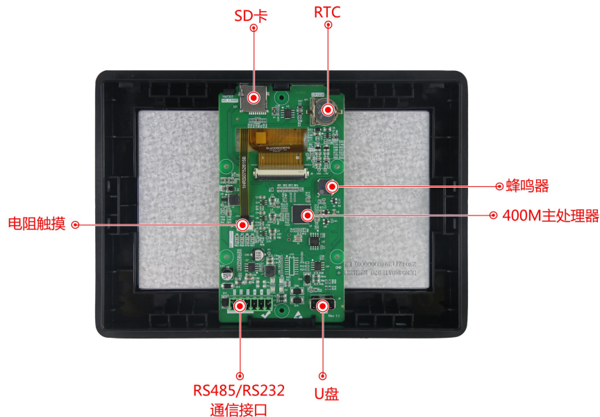
图 1-2 硬件配置图
